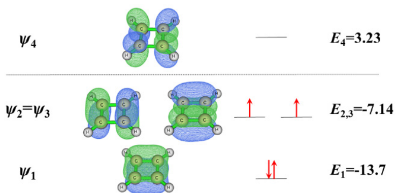
图 S1 环丁二烯离域 \pi 键分子轨道及能级图(eV)
